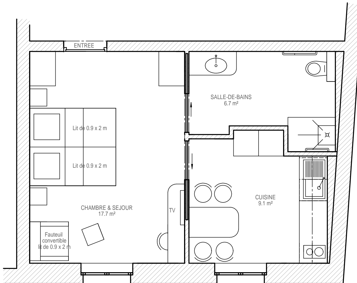
Implantation appartement Nord Ouest au rez-de-chaussée : adapté aux personnes à mobilité réduite
